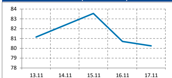
CO2-Preis (EEX EUA 2024)
