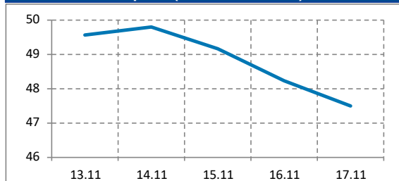
Gaspreis (PEGAS THE 2024)
