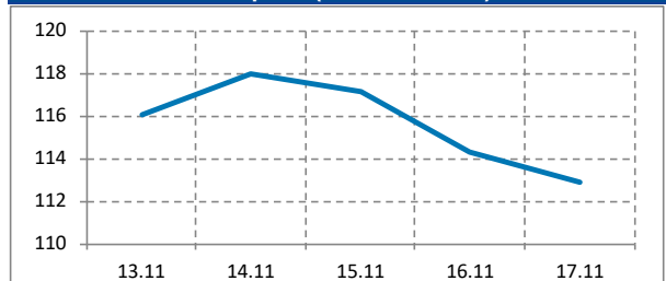
Strompreis (EEX Base 2024)
